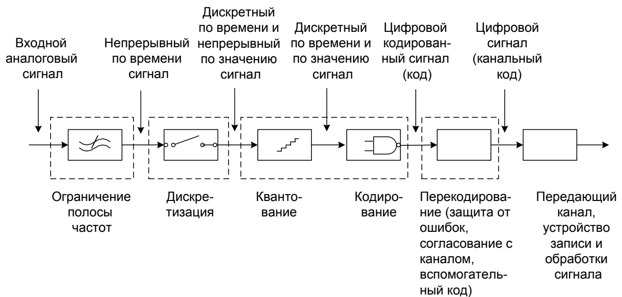
Рис. 4.1. Обобщенная структурная схема канала цифровой записи звука
