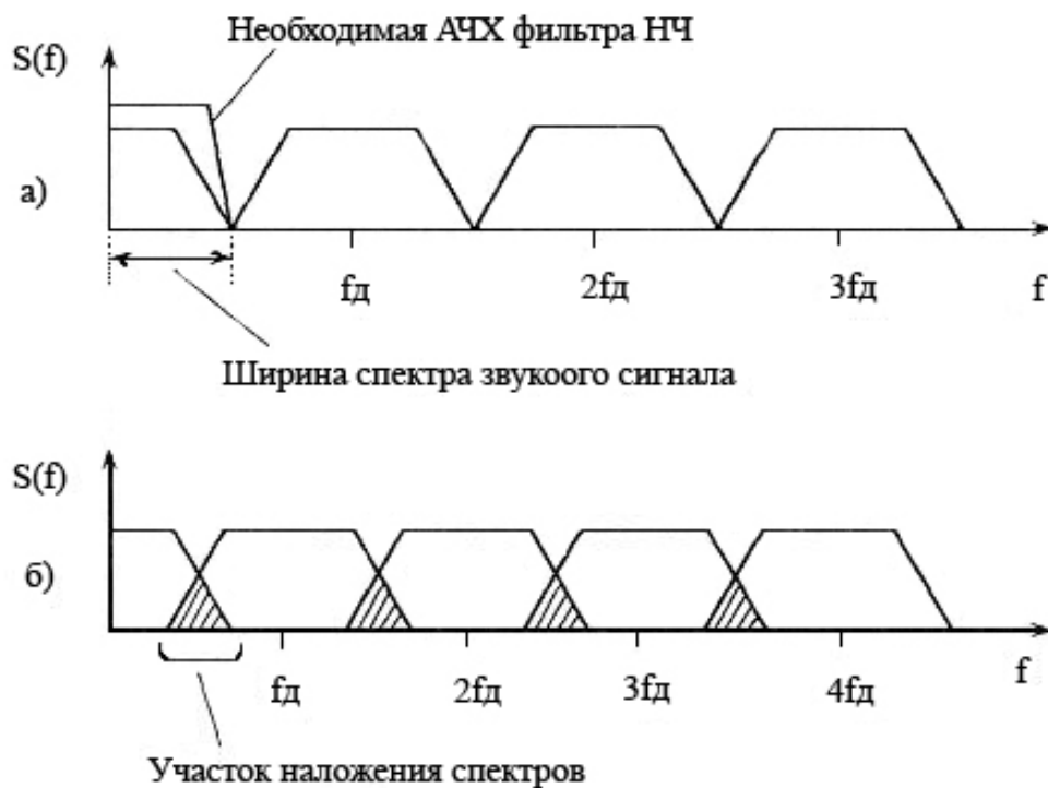
Рис. 4.2. Перекрытие спектров сигнала при дискретизации
